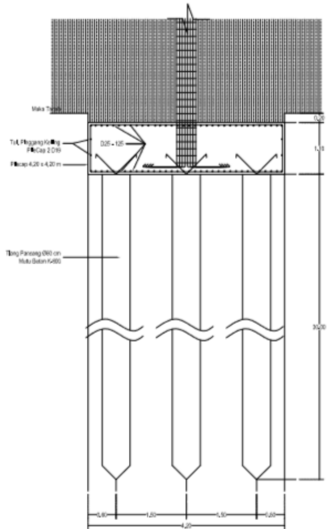
POTONGAN - C Skala 1:50
