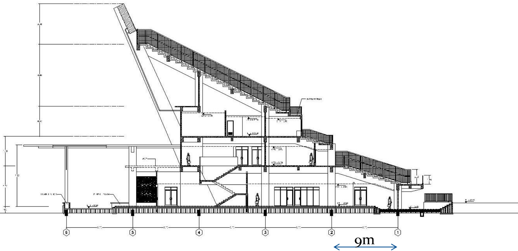
POTONGAN A-A SECTION 1 SKALA 1 : 150
